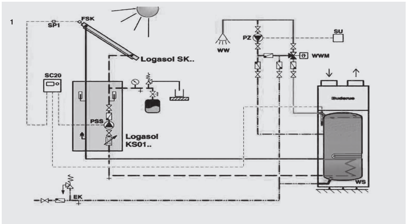
Εικ. 1 Αντλία θερμότητας για ζεστό νερό χρήσης σε συνδυασμό με ηλιακά και ανακυκλοφορία ζεστού νερού .
