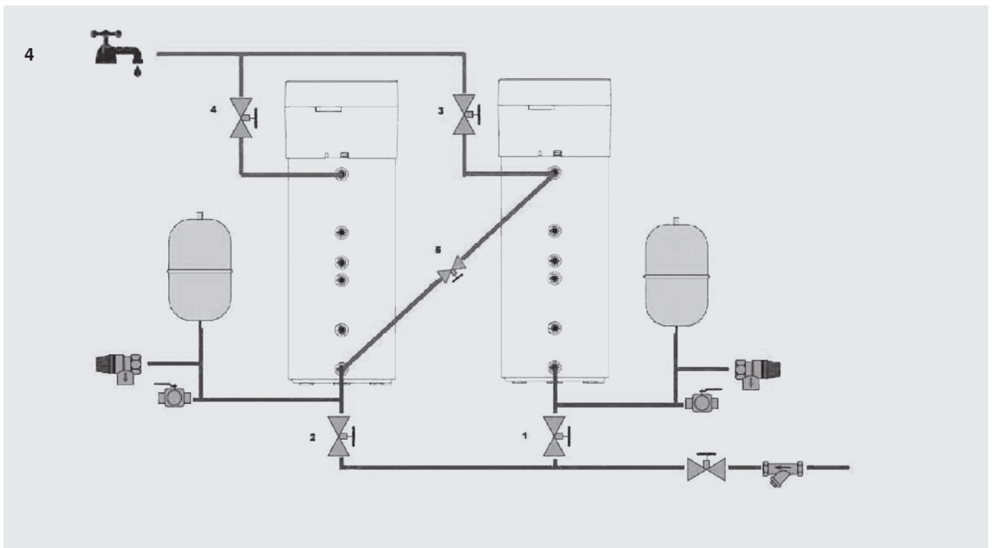
Εικ. 4 Παράλληλη σύνδεση αντλιών θερμότητας για ζεστό νερό αλλά με τη δυνατότητα να δουλέψουν σε σειρά.
