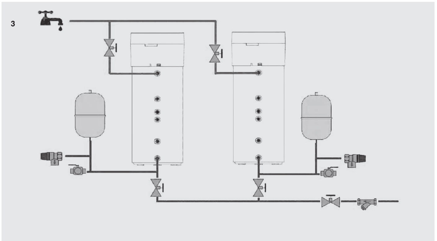
Εικ. 3 Παράλληλη σύνδεση αντλιών θερμότητας για ζεστό νερό
