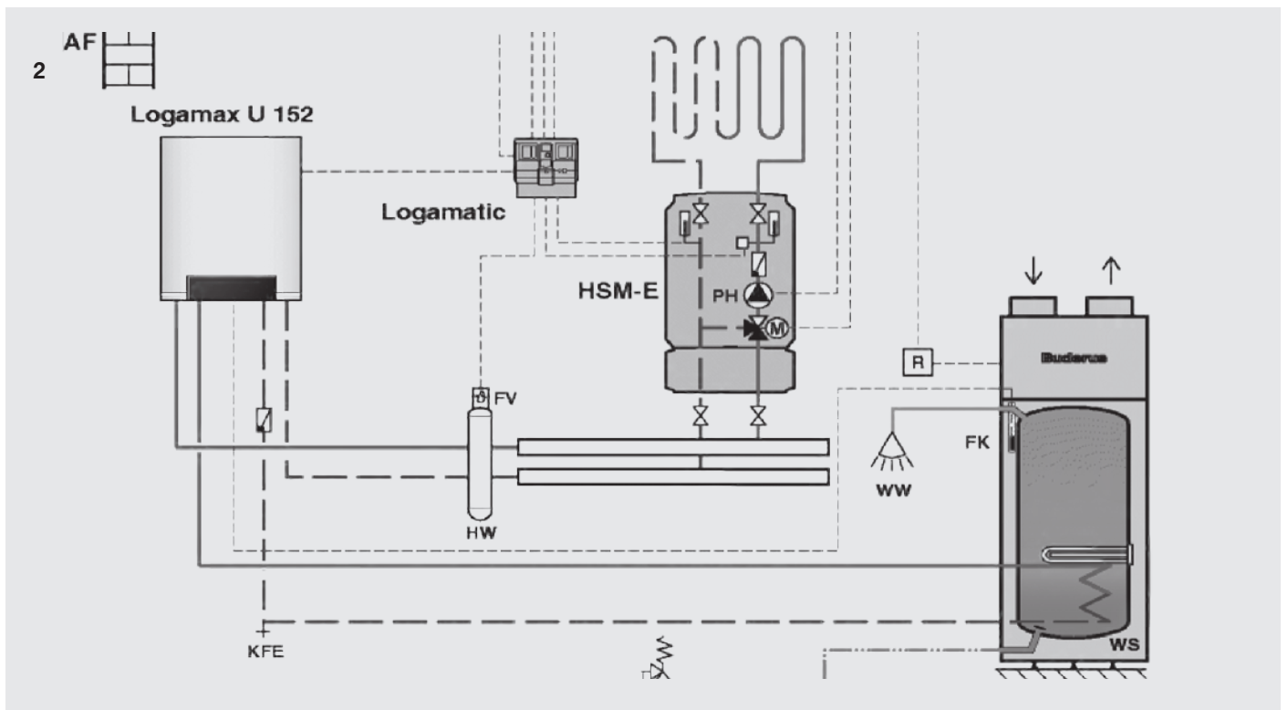
Εικ. 2. Αντλία θερμότητας για ζεστό νερό χρήσης σε συνδυασμό με λέβητα αερίου
